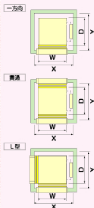
昇降機平面図
