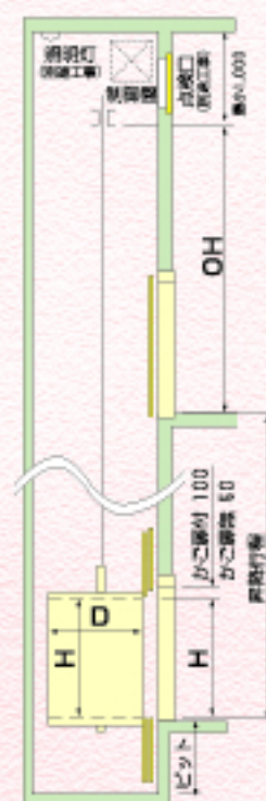
昇降面断面図
